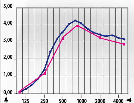
Schallabsorptionsgrad DIN EN 20354 Sound absorption ISO 354
